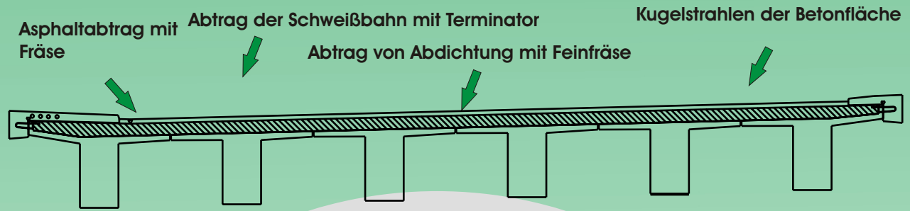
Abschälen der Schweißbahn mit dem Terminator - die Betonoberfläche wird kaum beschädigt - im günstigsten Fall reicht Kugelstrahlen als weiterer Arbeitsschritt
